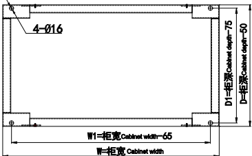
FS柜活动底座示意（固定同） FS cabinet base to indicate activity (fixed with)
